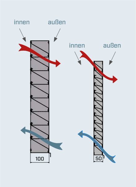
Schnitt LLE Aluminiumlüfter Bautiefe 100 mm Bautiefe 50 mm
