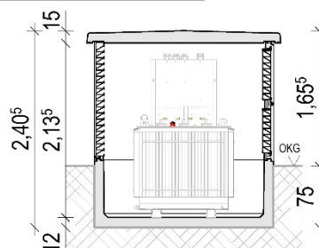
Querschnitt M 1 : 50
