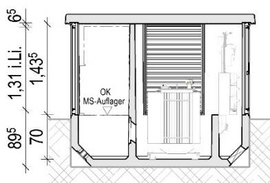
Längsschnitt M 1 : 50
