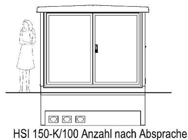
Ansicht D
