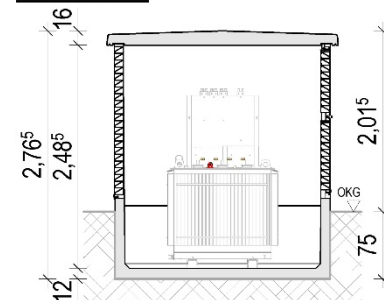
Querschnitt
