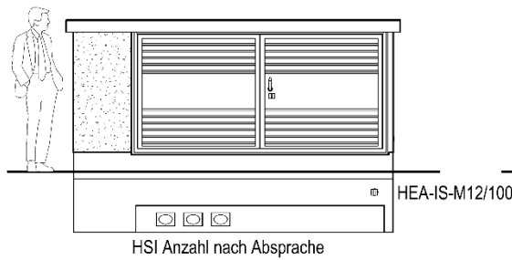
Ansicht C
