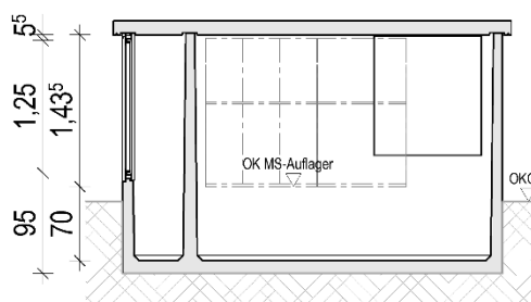
Längsschnitt
