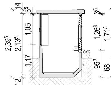
Querschnitt
