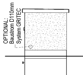
Ansicht D
